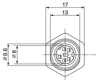
TCS7392(Socket)
