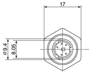
TCP7391(Plug)
